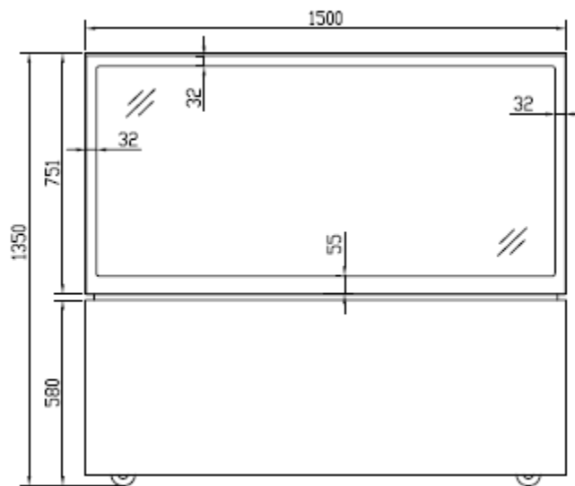
ELEVATION 前视图
