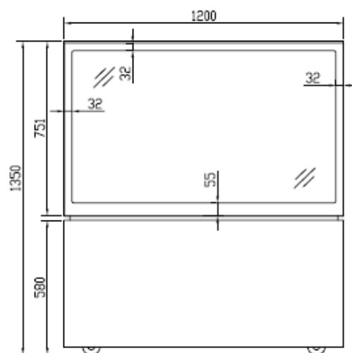
ELEVATION 前视图
