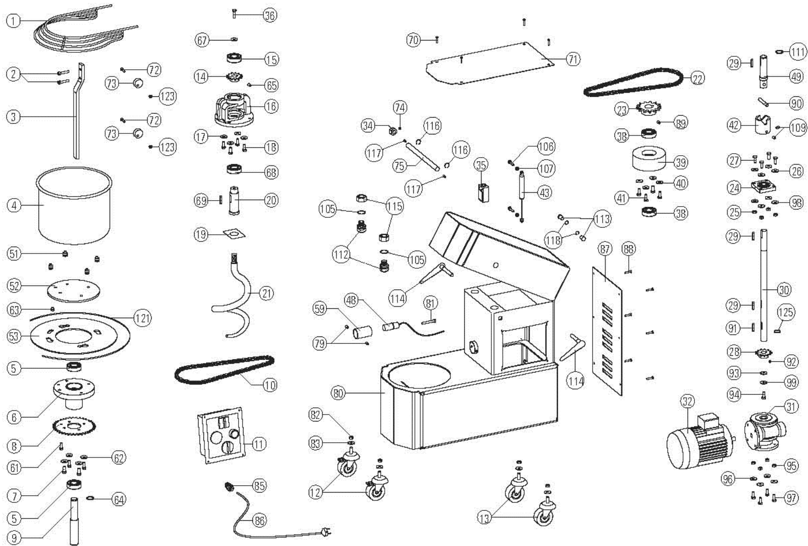
FIG. 22 Pièces de rechange pour pétrisseuse avec tête soulevable et cuve extractible mod. IM 25-38-44 A BILD 22 Ersatzteile für die Teignet-maschine mit hebbarem Kopf und herausziehbarem Becken mod. IM 25-38-44 A
